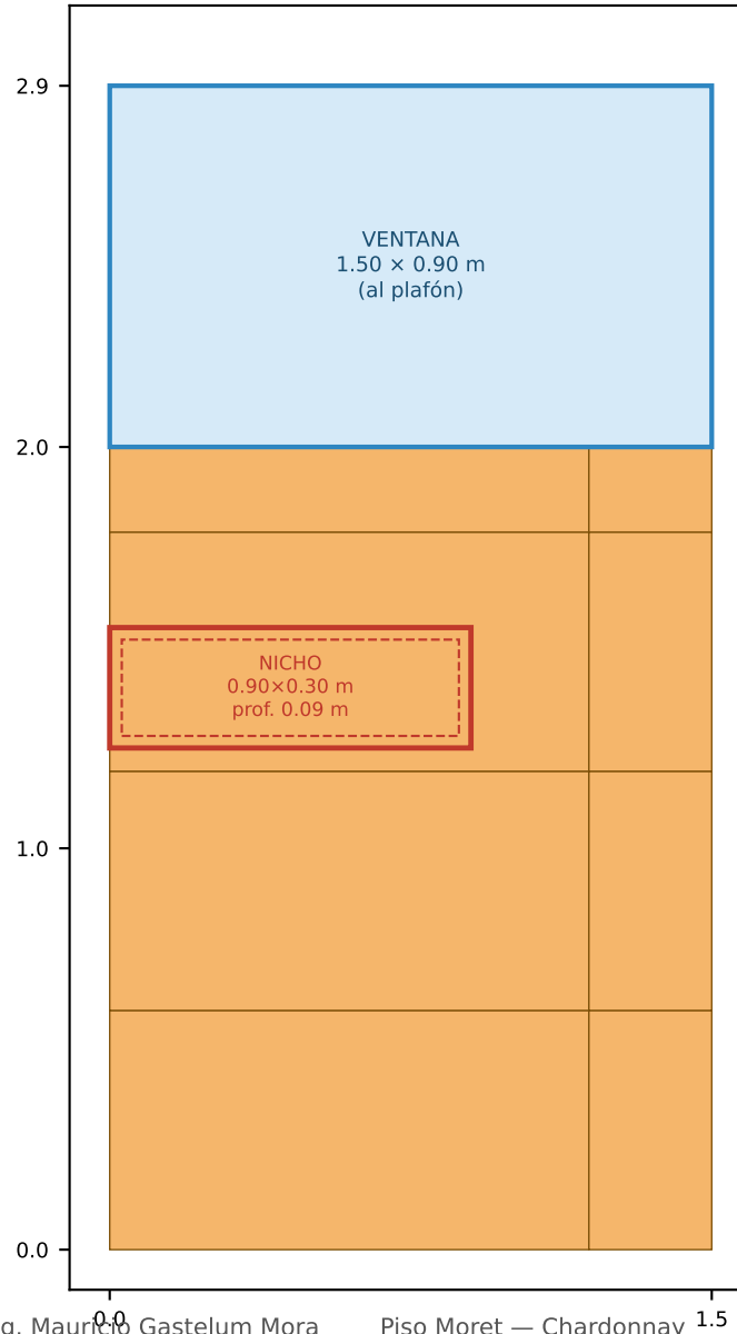
Regadera 2 (P.A.) muro de fondo 1.50 × 2.90 m 3 caras – ventana = 9.96 m 2
